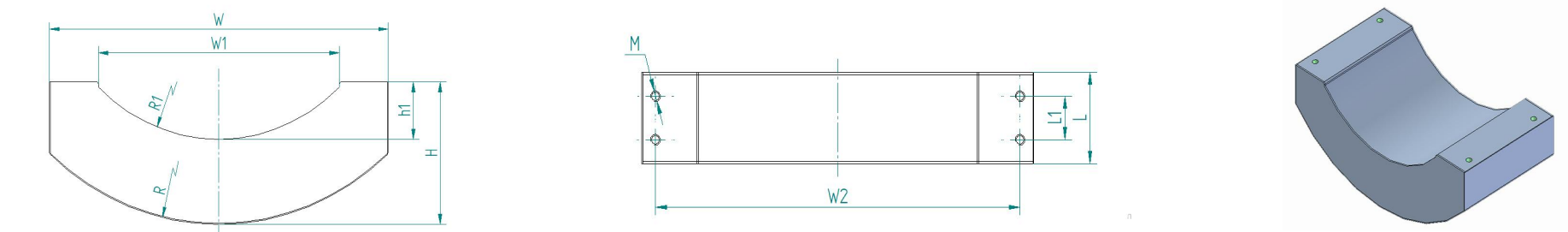
R系列磁力瓦参数表 The parameter table of R series magnetic wheel(NdFeB)
